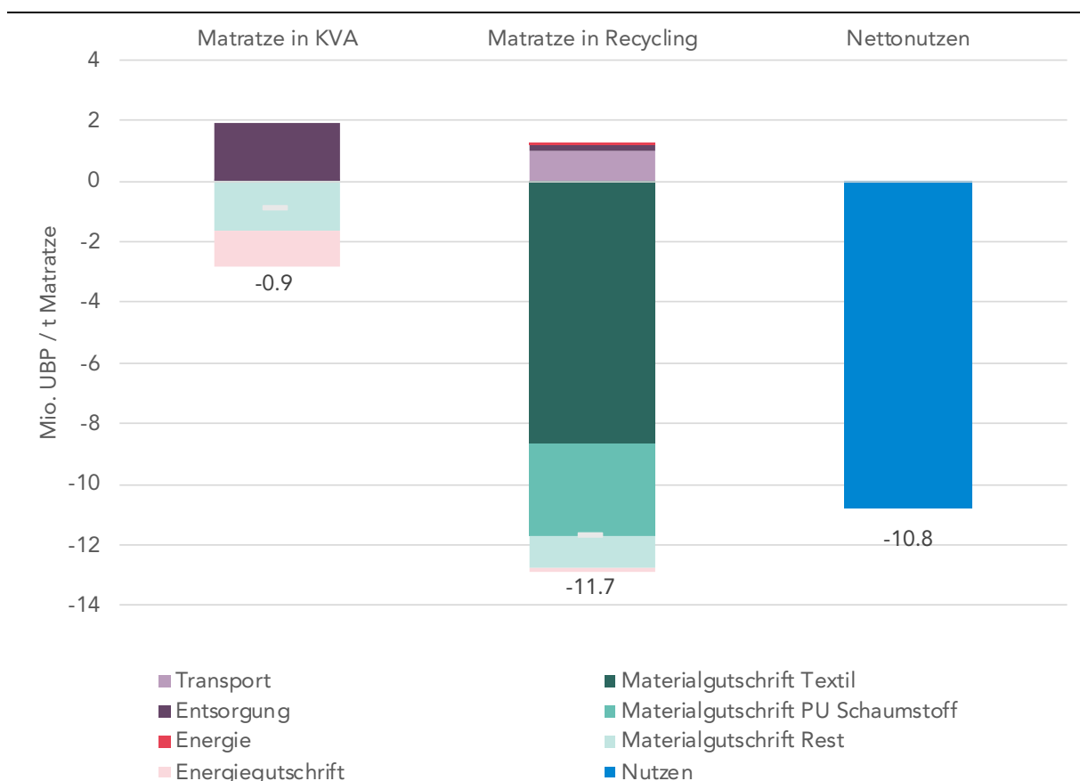
Abbildung 7: Umweltfussabdruck der beiden Matratzenverwertungen sowie Nettonutzen UBP: Methode der ökologischen Knappheit 2021
