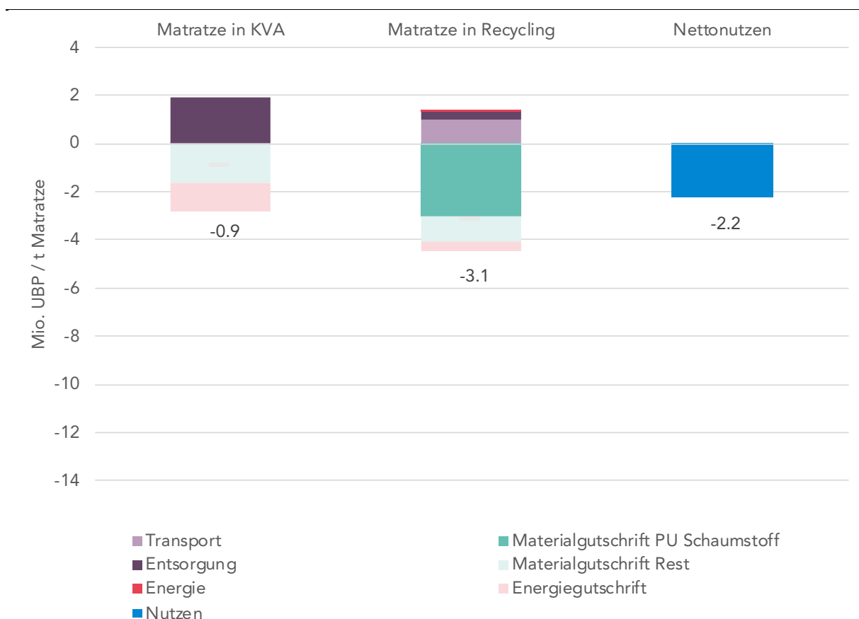
Abbildung 9: Umweltfussabdruck der beiden Matratzenverwertungen sowie Nettonutzen
