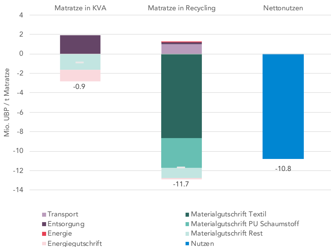
Abbildung 2: Umweltfußabdruck der beiden Matratzenverwertungen sowie Nettonutzen
