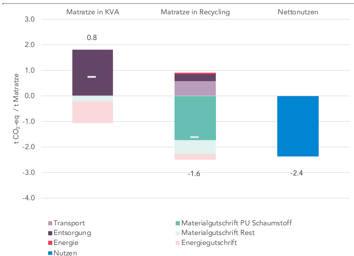
Abbildung 8: CO 2 -Fussabdruck der beiden Matratzenverwertungen sowie Nettonutzen CO 2 -eq: IPCC 2021 (GWP100)
