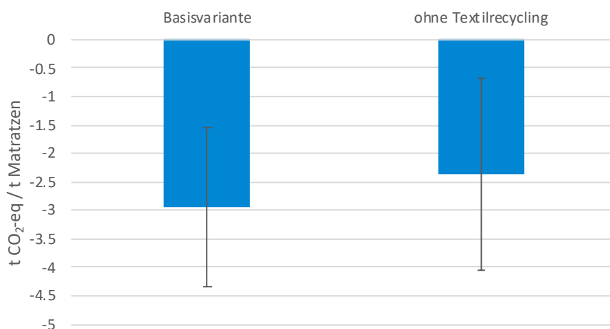
Abbildung 10: MC-Analyse (1000 runs): Darstellung der Unsicherheit auf dem 95% Niveau (in 95 % aller berechneten Fälle liegt der Nutzen innerhalb des Fehlerbalkens)
