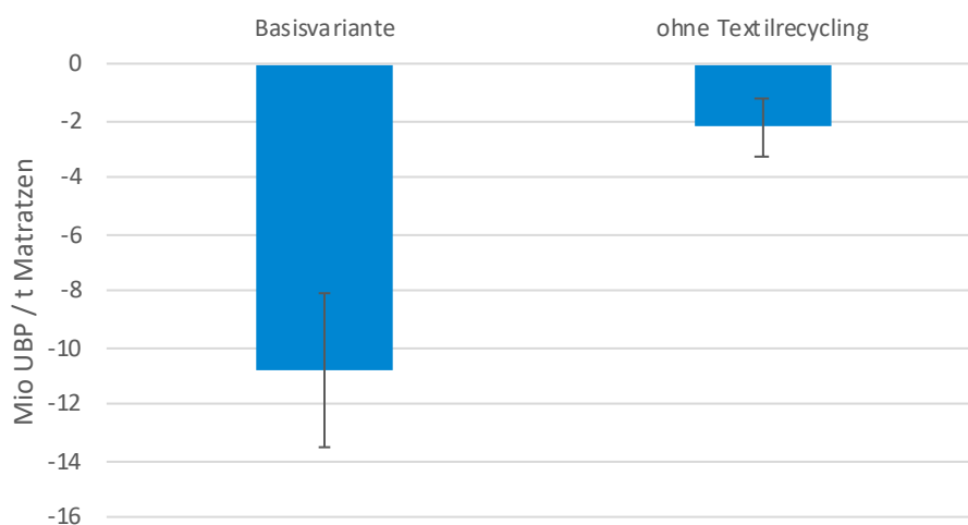
Abbildung 11: MC-Analyse (1000 runs): Darstellung der Unsicherheit auf dem 95% Niveau (in 95 % aller berechneten Fälle liegt der Nutzen innerhalb des Fehlerbalkens)
